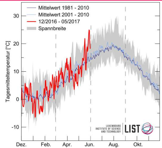
Gemittelter Jahresgang (2001 – 2010 hellblau; 1981 – 2010 dunkelblau) der Lufttemperatur im Vergleich zu dem Zeitraum 12/2016 bis 05/2017 (rot). Die Spannbreite ist definiert durch die absoluten Minima und Maxima der Tagesmitteltemperatur (grau). Datenquelle: Rohdaten MeteoLux (Station Findel).
