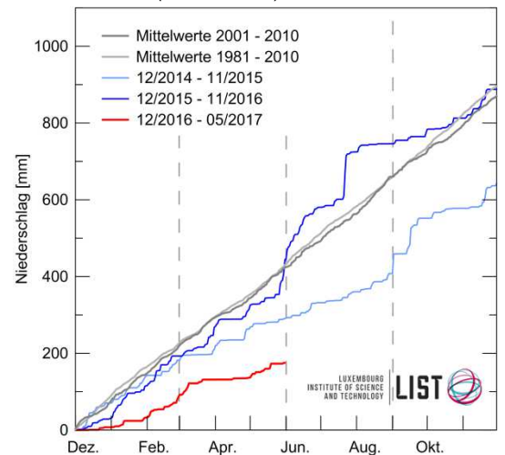
Gemittelte Niederschlagssummen (2001 – 2010 schwarz; 1981 – 2010 grau) im Vergleich zu dem Zeitraum 12/2016 bis 05/2017. Datenquelle: Rohdaten MeteoLux (Station Findel).
